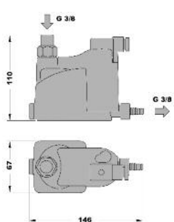
ED3002 0,5 kg
