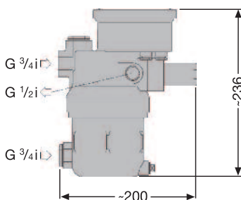
ED2020 2,9 kg
