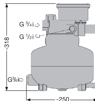
ED2060 9,4 kg
