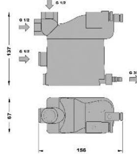
ED3030 1,1 kg
