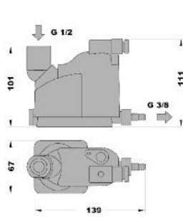
ED3004 0,6 kg
